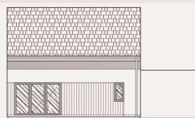
ELEWACJA TYLNA
