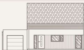
ELEWACJA FRONTOWA
