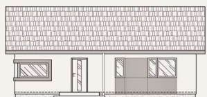
ELEWACJA FRONTOWA
