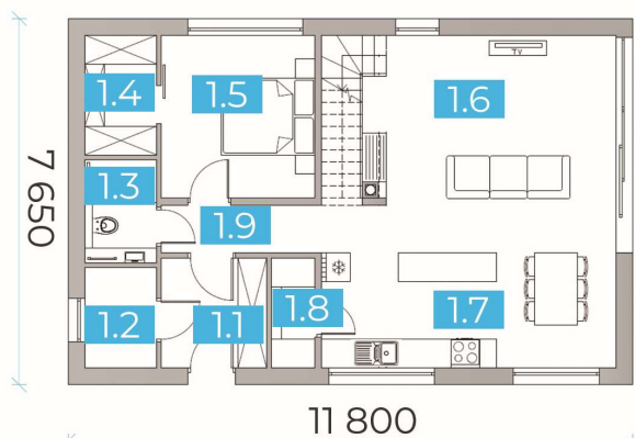
RZUT PARTERU
