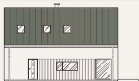
ELEWACJA FRONTOWA
