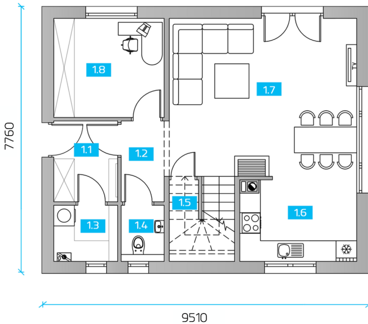
RZUT PARTERU
