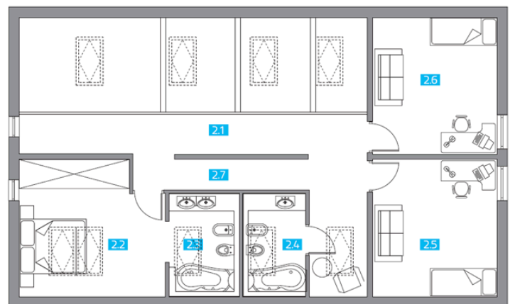
RZUT PODDASZA
