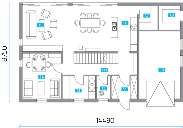
RZUT PARTERU
