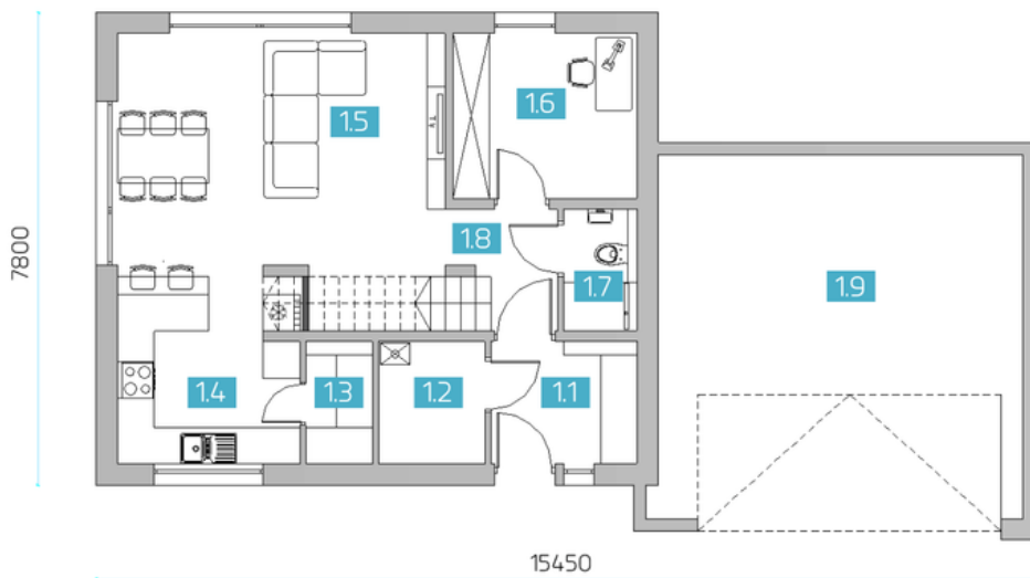
RZUT PARTERU
