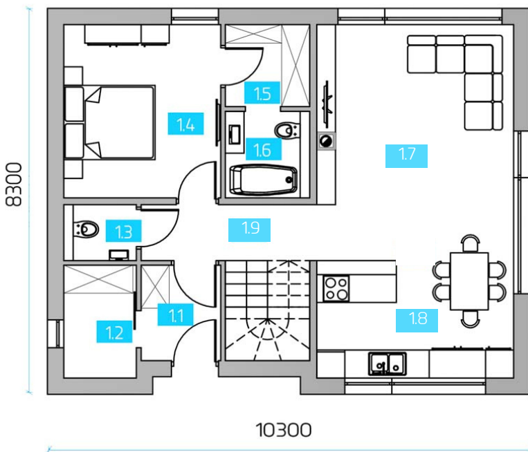
RZUT PARTERU
